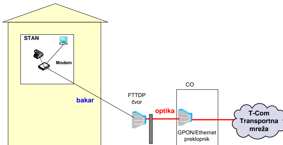
Slika 36. Način realizacije FTTDP koncepta u pristupnoj mreži
