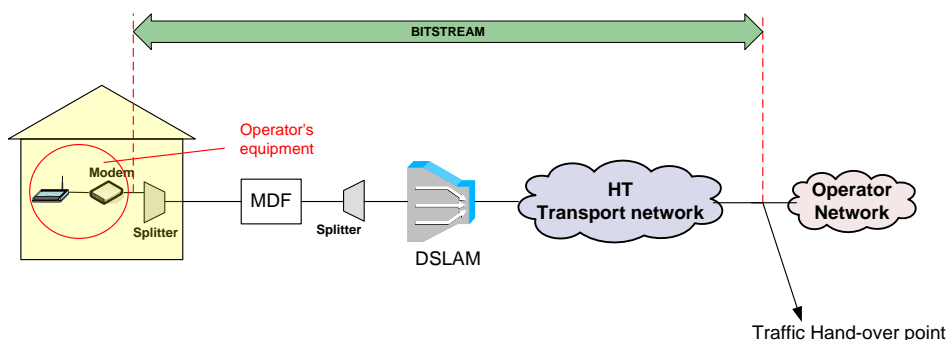
Slika 32. Koncept posebnog virtualnog kanala za Podatkovnu uslugu
