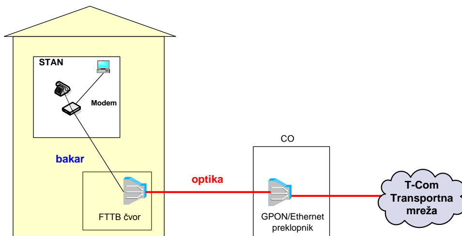
Slika 35. Način realizacije FTTB koncepta u pristupnoj mreži
